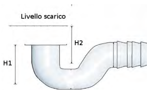
Scarico condensa laterale
